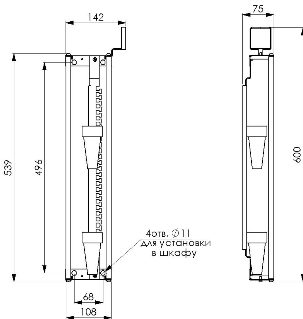
Рис.2 Габаритный чертеж бокса кабельного
